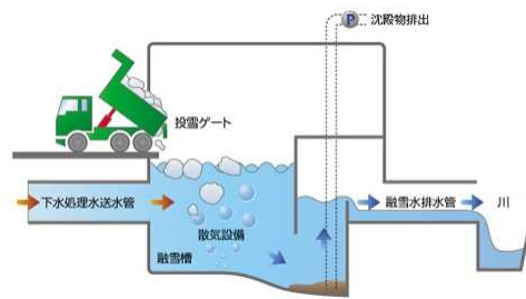
(例)下水廃熱を利用した融雪設備
