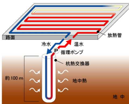
(例)地中熱ロードヒーティング
