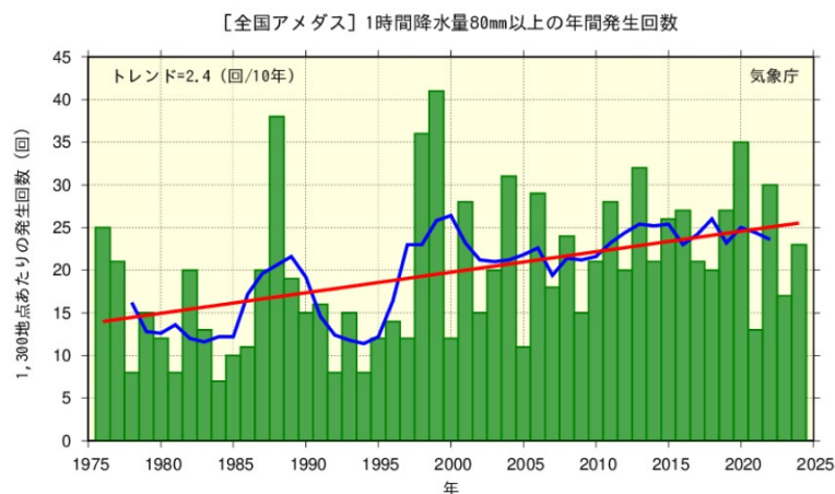
図 1 1時間降水量 80 ミリ以上の年間発生回数（1976 年から 2024 年）
