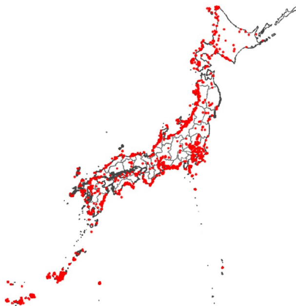
図 竜巻分布図（1961～2024 年）
